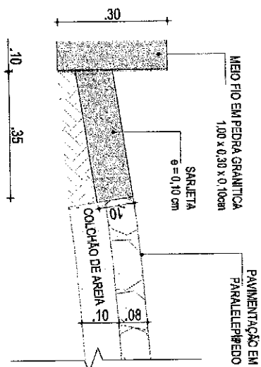
03 | DETALHE - MEIO FIO PEDRA GRANITICA E SARJETAS ESQ: 1/10
