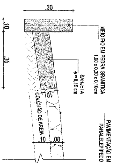
03 DETALHE - MEIO FIO PEDRA GRANITICA E SARJETAS
